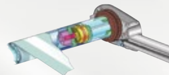
Λεπτομέρεια του ομοαξονικού συστήματος Coaxial Technique
